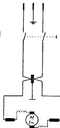
WIRING-DIAGRAM SCHALTPLAN
