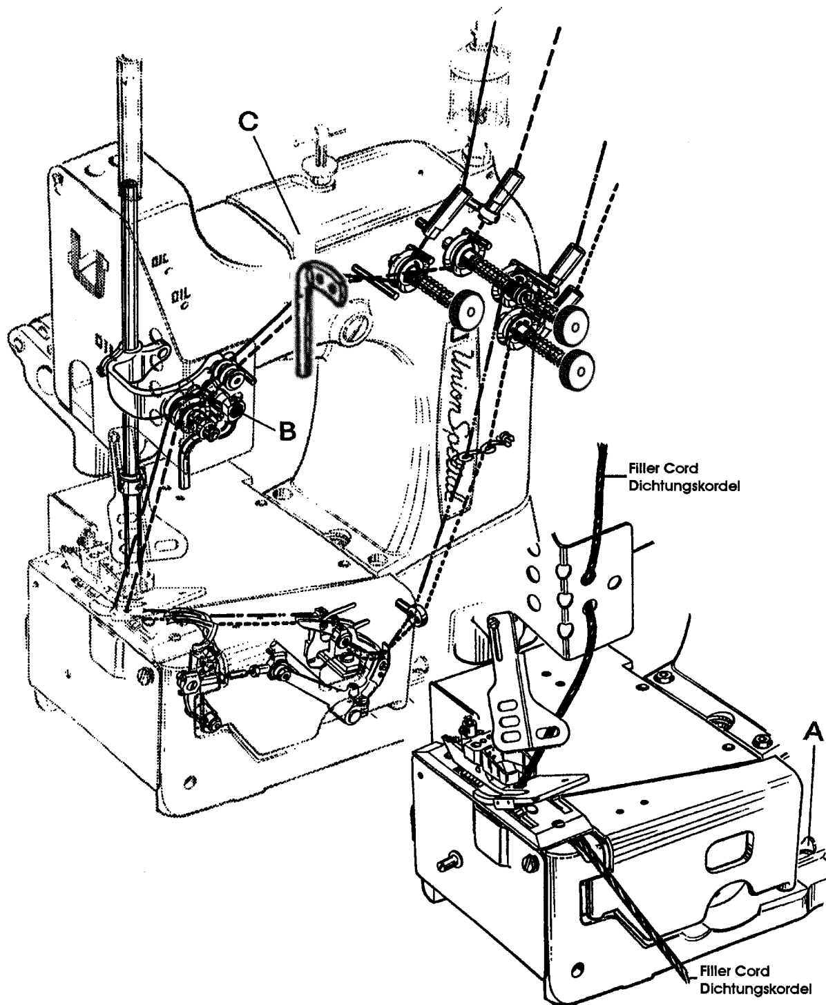
THREADING DIAGRAM FOR STYLES 80700CD3, CD4, CD4HLU EINFÄDELANLEITUNG FÜR DIE TYPEN 80700CD3, CD4, CD4HLU
