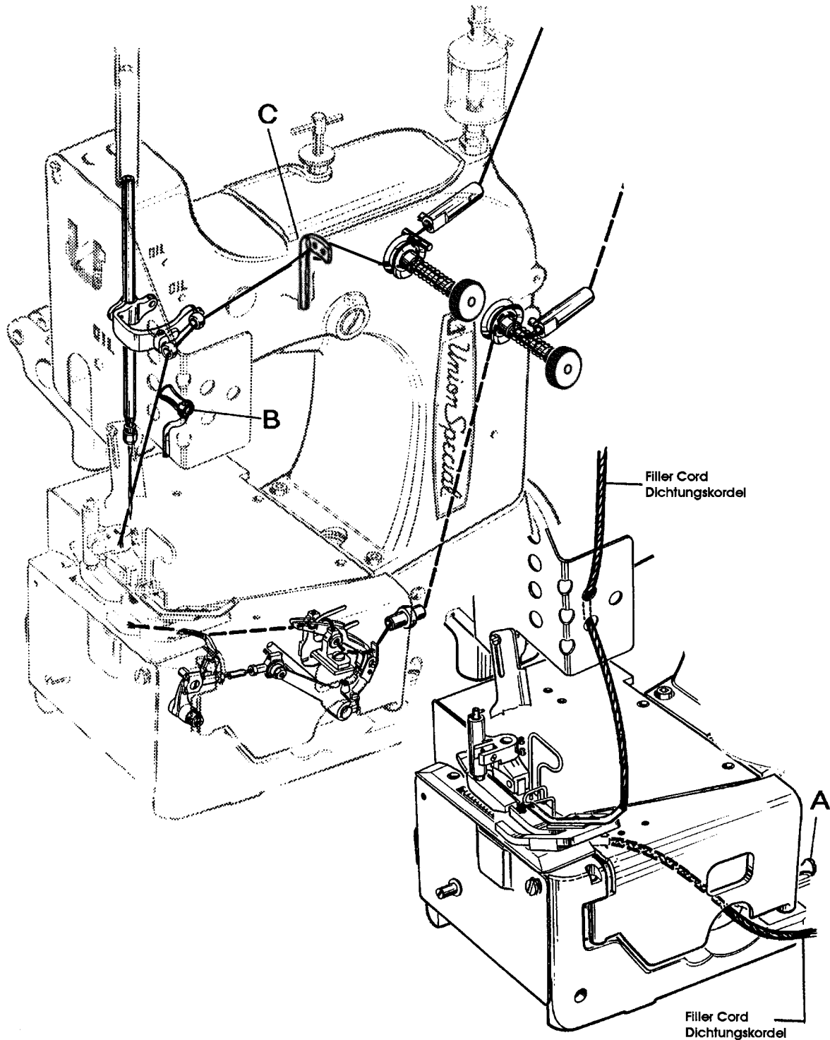
THREADING DIAGRAM FOR STYLES 80700C3, C4, C4HLU EINFÄDELANLEITUNG FÜR DIE TYPEN 80700C3, C4, C4HLU
