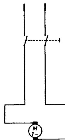
WIRING-DIAGRAM SCHALTPLAN
