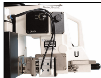
Umschlag-Verschluss von Hand durch Bediener oder durch zusätzliche Sackzuführeinrichtung mit Sackumfaltenrichtung
