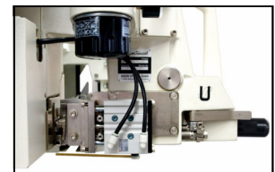
Nähen ohne Reiterband
