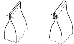
Umschlag-Verschluss von Hand durch Bediener oder durch zusätzliche Sackzuführeinrichtung mit Sackumfalteinrichtung
